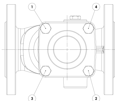
Kolejność dokręcania śrub łączących Kadłub z pokrywą
