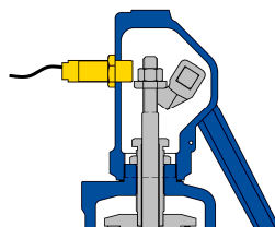
Wykonanie z czujnikiem zadziałania
