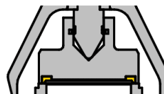
Wykonanie z doszczelnieniem miękkim (-2, -3)
