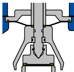
Wykonanie z membraną (01-4)
