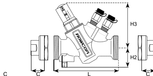
Model zaworu ABV z kartridżem E-JUST
